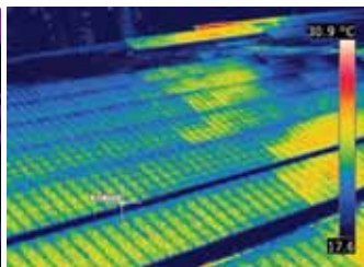
Esta termografía muestra grandes zonas con temperaturas elevadas. Sin más información, no se percibe si estas anomalías son térmicas o provocadas por ensombrecimientos/reflejos.
