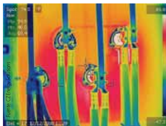
Las cámaras termográficas también se pueden utilizar para examinar el sistema completo que rodea a las turbinas eólicas. Uno de estos conectores de tres fases, el del extremo derecho, está mucho más caliente que el resto. Este defecto se detectó y pudo repararse antes de que provocara una avería.
