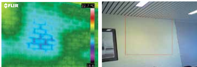
Falta aislamiento en partes del muro.
