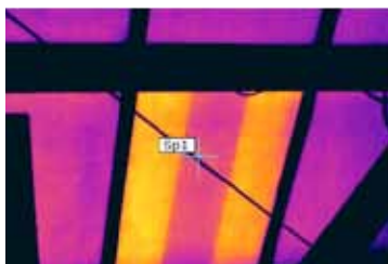
Dos hileras de celdas aparecen calientes en la termografía, lo que indica que hay diodos de derivación rotos.
