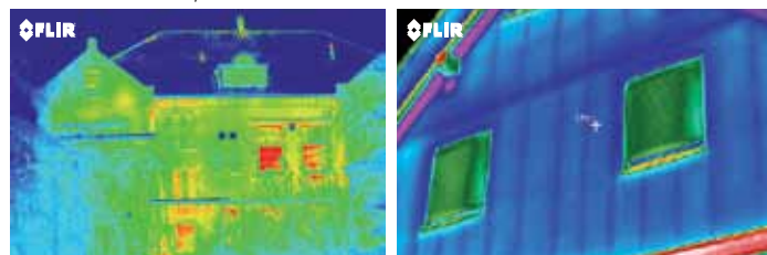
Inspección térmica desde el exterior, las termografías indican claramente falta de aislamiento o aislamiento defectuoso.
