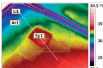
Con una cámara termográfica podrá localizar rápidamente problemas como celdas dañadas y así resolverlos de manera rápida.
