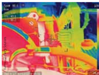
Termográfica para inspección de turbina eólica. Esta inspección tuvo lugar a una altura de unos 50 metros.
