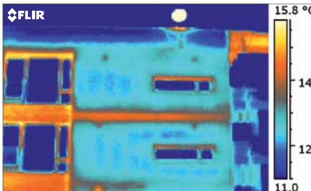
La imagen muestra un puente término en uno de los pisos.
