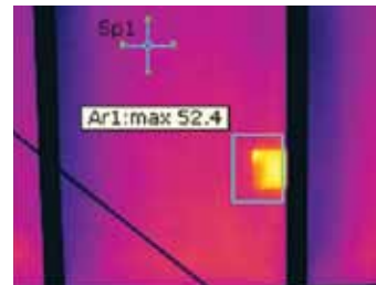
Esta termografía muestra un punto caliente provocado por la rotura de celdas en una placa estándar de 60 celdas.
