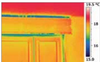
Termografía
