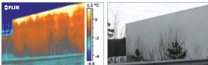
Almacén con gran cantidad de aire caliente saliendo entre la pared y el tejado. Estas uniones deben ajustarse para evitar la pérdida de energía.
