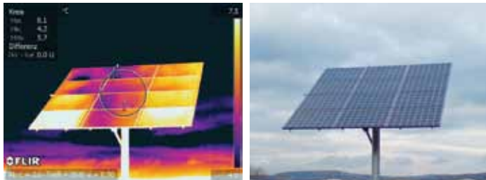
Los puntos calientes de esta termografía tomada de la parte delantera del panel solar parecen indicar que muchas celdas no funcionan de forma eficaz.
